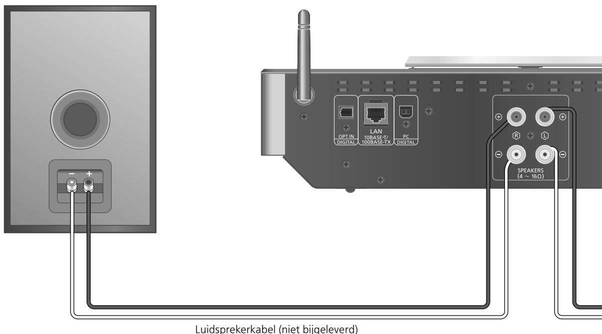
Luidsprekerkabel (niet bijgeleverd)
