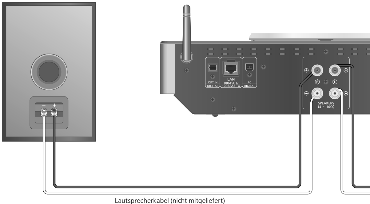
Lautsprecherkabel (nicht mitgeliefert)
